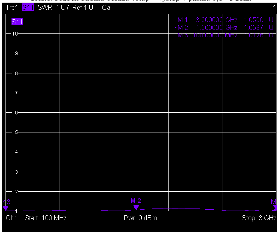
Graf.2. Průběh PSV vstup – výstup v pásmu 0,1 –3 GHz.
