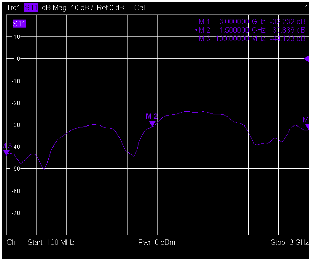
Graf.1. Průběh útlumu odrazu vstup – výstup v pásmu 0,1 - 3GHz.
