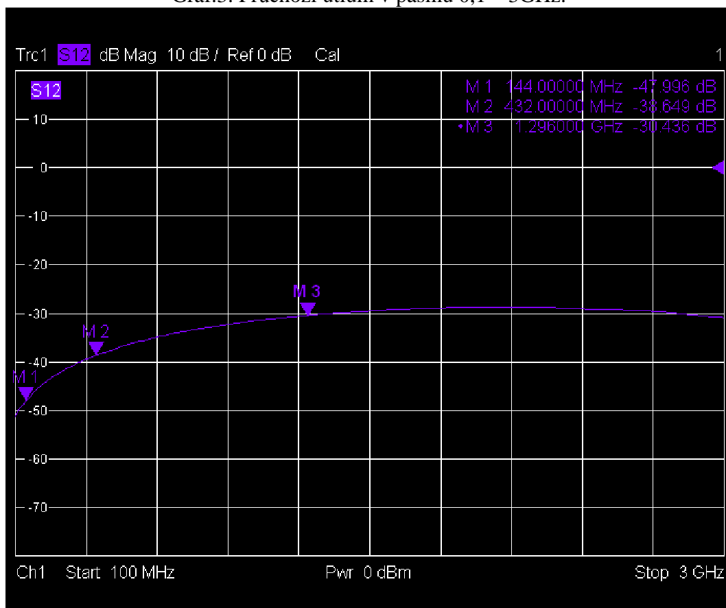
Graf.5 Průběh útlumu směrové vazby v pásmu 0,1 – 3GHz.
